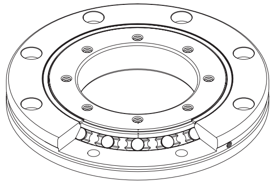
Model RU
