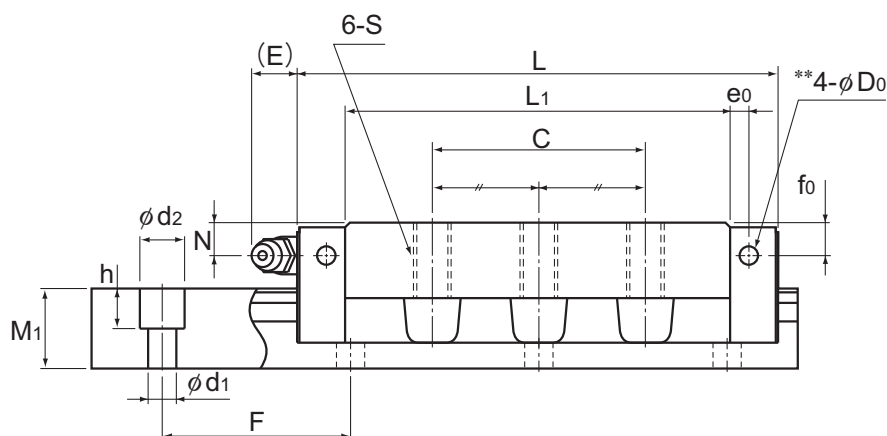
Model NR-LA
