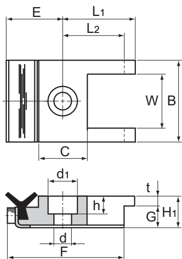
Model SE
