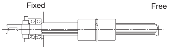
Fixed - free
