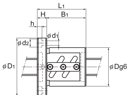
Model BNF
