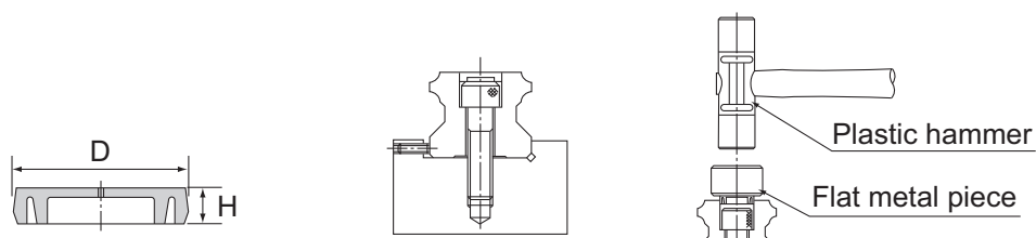
Fig.1 Cap C
